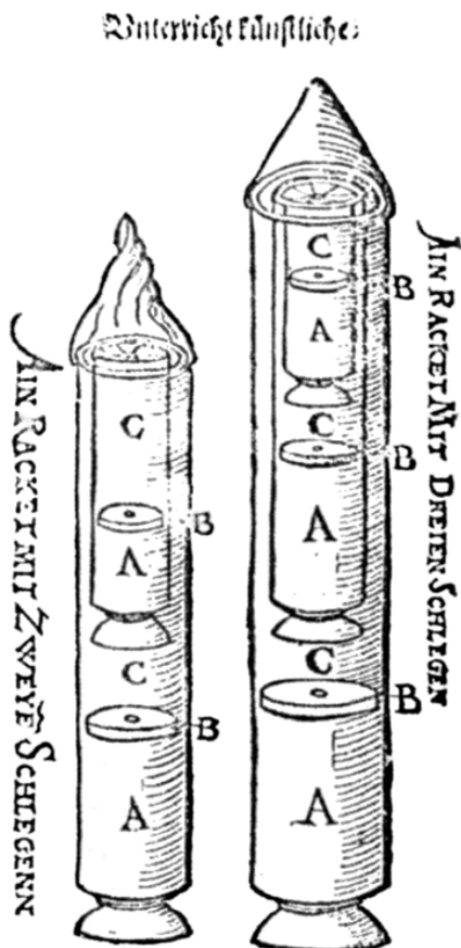
Conrad Haas (1529 – 1569), „Königlicher und Kaiserlicher Zeugmeister“ in Hermannstadt. Entwurf, „Wie du solt machen gar schöne Rackette, die da von im selber oben hienauß in die hoch faren“.
