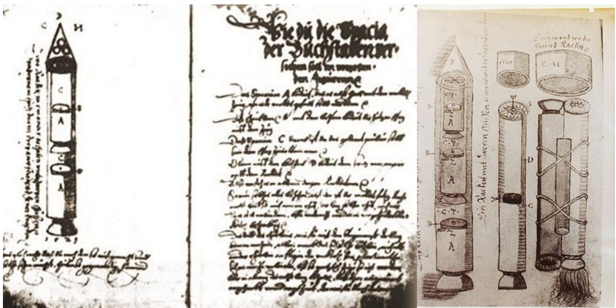
Conrad Haas (1529 – 1569), „Königlicher und Kaiserlicher Zeugmeister“ in Hermannstadt. Entwurf, „Wie du solt machen gar schöne Rackette, die da von im selber oben hienauß in die hoch faren“.
